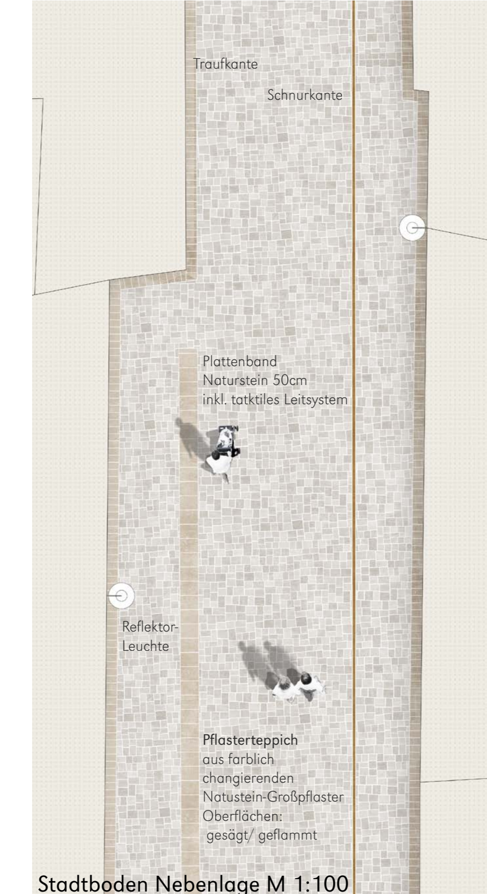
Stadtboden Nebenlage M 1:100
